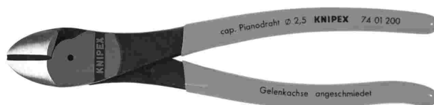
Kraftseitenschneider | Pianodraht
